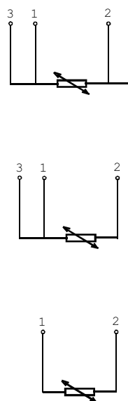
Схематичне зображення з'єднань
