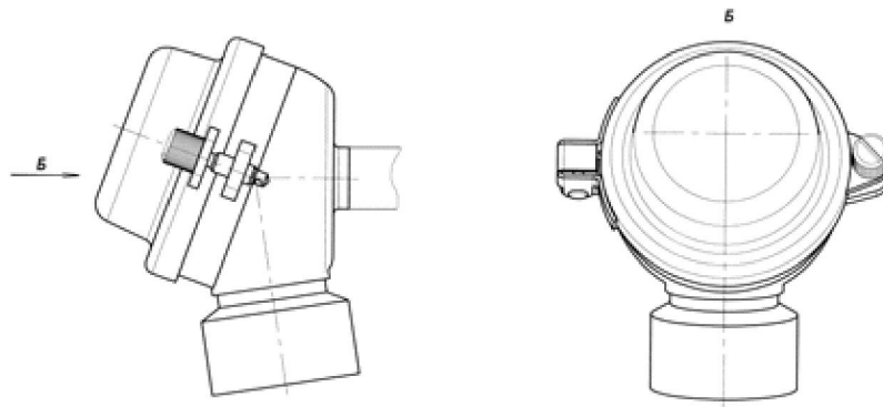
Рис. 8 - Чертеж наружной части ТХА-1090, ТХК-1090 с головкой типа БАУИ.408724.023 СБ
