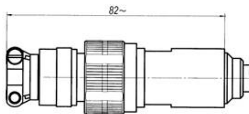
Рис. 9 - Кресленик зовнішньої частини ТХА-1090, ТХК-1090 з головкою БАУИ.408724.025 СБ
