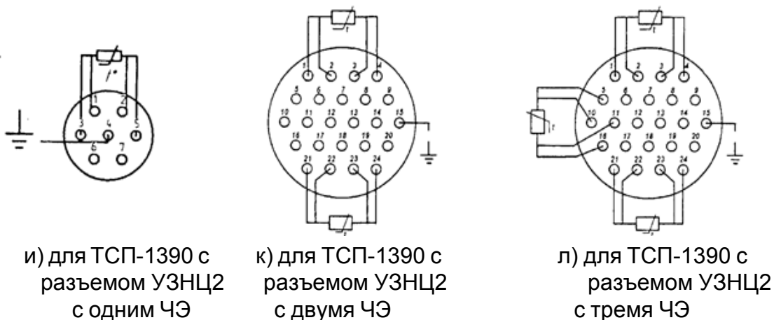
Рис. 2 - Электрические схемы подсоединения ТСП-1390 с разъемом
