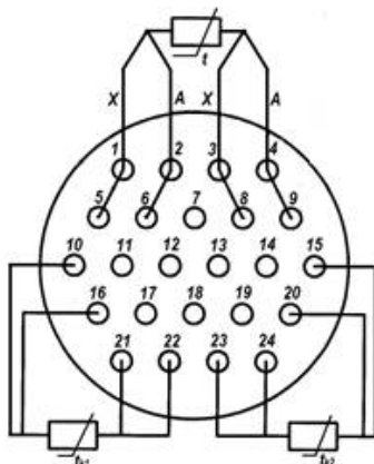
Рис. 4 - Электрические схемы подсоединения ТСП-1390 с разъемом в комплекте с ТХА-1690 с встроенными ЧЭ
