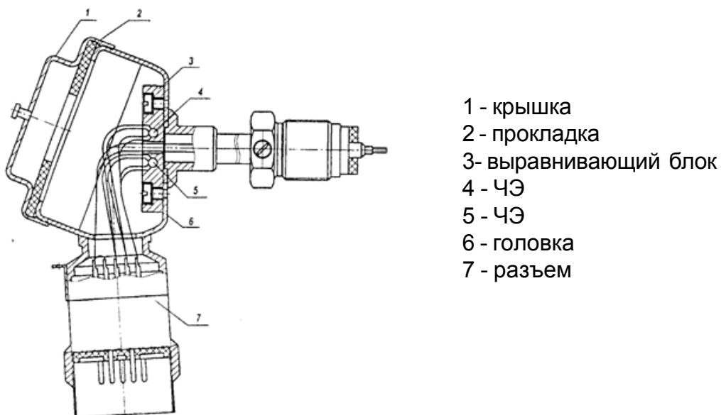
Рис. 3 - Чертеж наружной части ТСП-1390 с разъемом в комплекте с ТХА-1690 с встроенными ЧЭ
