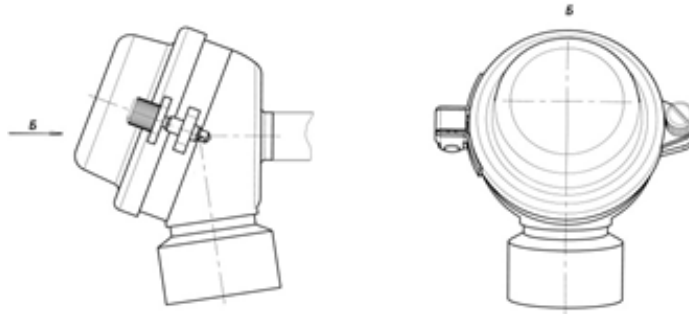
Рис. 7 - Кресленик зовнішньої частини ТСП-1390 з головкою БАУИ.408724.023 СБ
