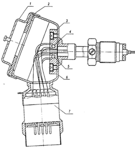
Рис. 3 - Кресленик зовнішньої частини ТСП-1390 зі з'єднувачем у комплекті з ТХА-1690 з вмонтованими ЧЕ
