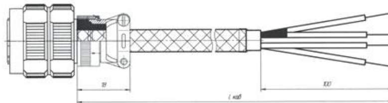
Рис.10 - Кабельная линия связи MULTITHERM 400-ES с разъемом УСНЦ144 для режима ТА
