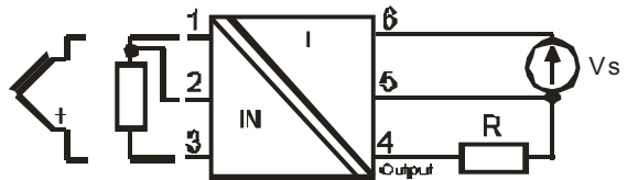
Рис. 3 - ПВП-0205, ПВП-0305
