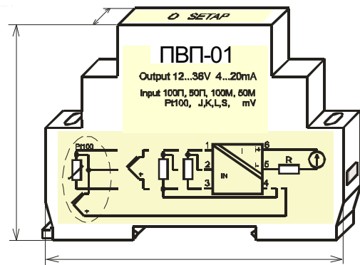
Рис. 1 - ПВП-01
