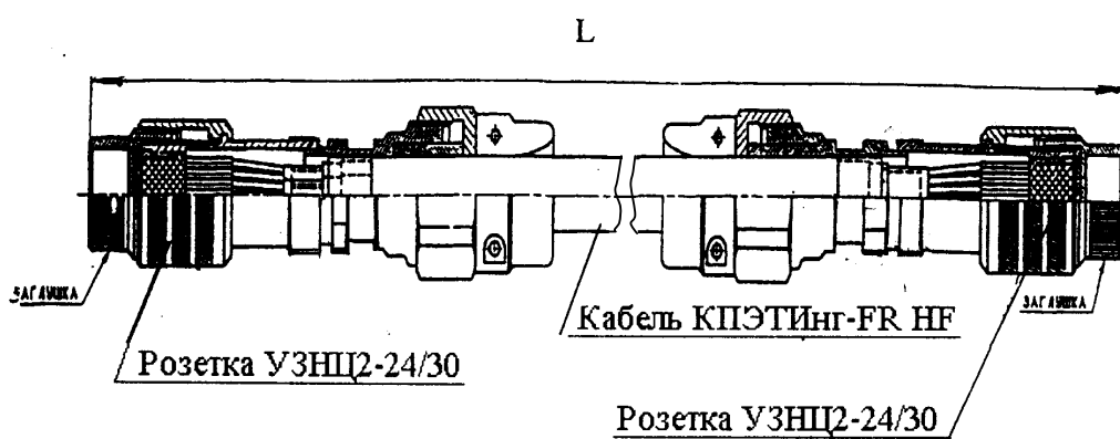
Рис. 1 - Габаритний кресленик джгутів ТК
