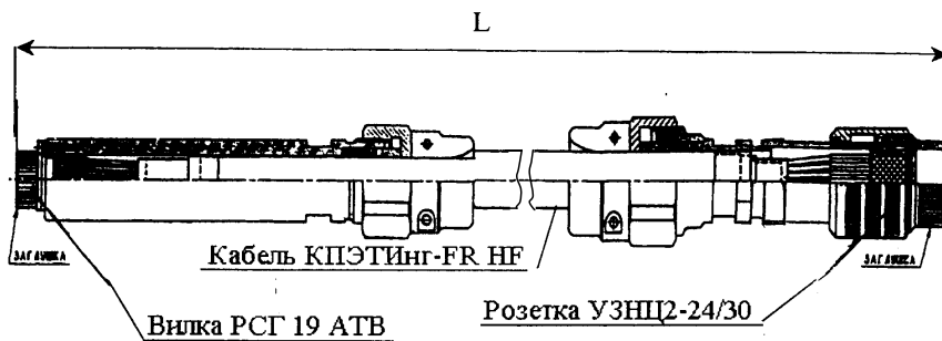
Рис. 2 - Габаритний кресленик джгутів EB
