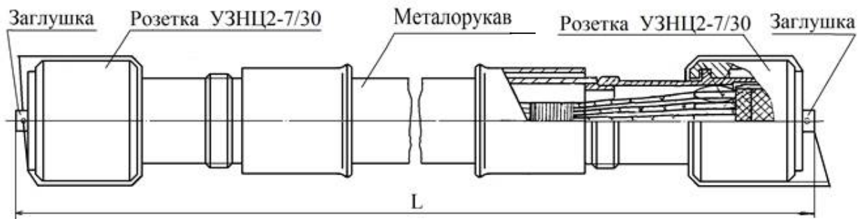
Рис. 4 - Габаритний кресленик джгутів ЕМ*
