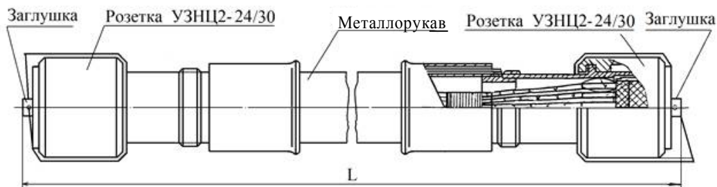
Рис. 5 - Габаритний кресленик джгутів ДП*
